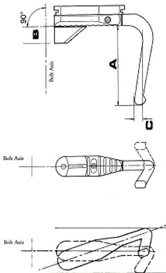
Slika 326-3 Dimenzijske omejitve ramenske kljuke
